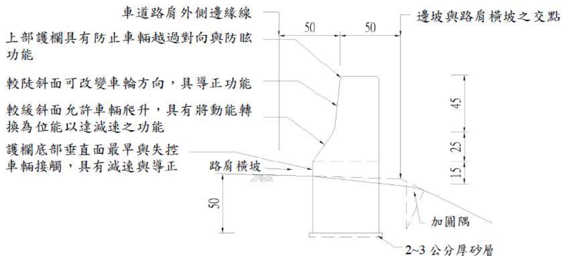
剖面圖
